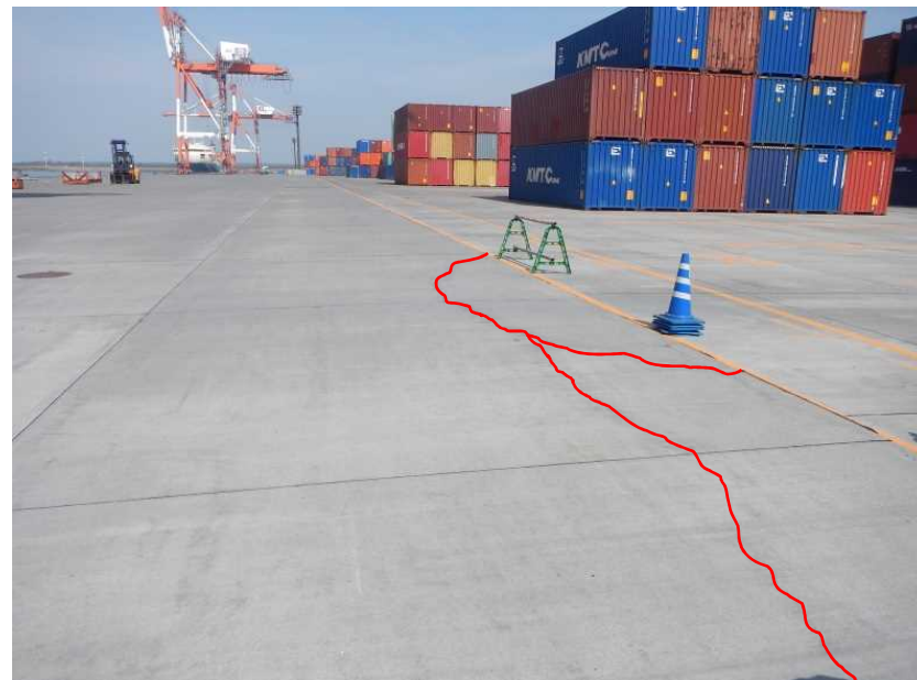
中央ふ頭2号岸壁 エプロンひび割れ
