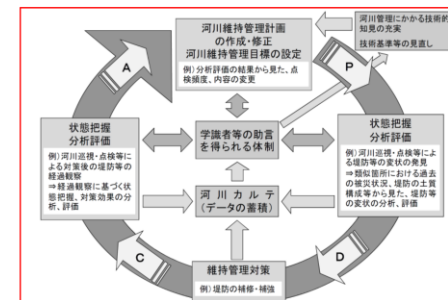
図 2-8 サイクル型維持管理体系のイメージ
