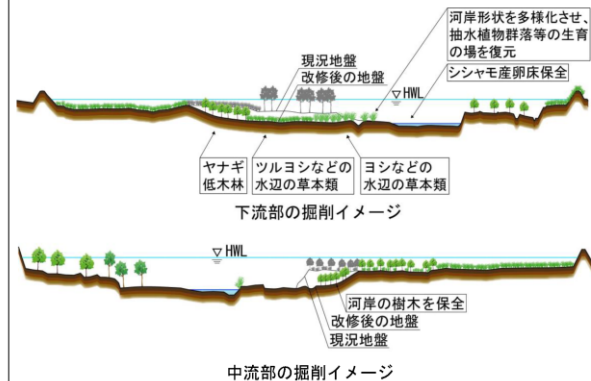
図 2-1-7 流下能力不足により対策が必要な断面横断面図
