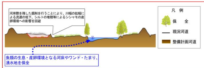
図 2-7 河道掘削のイメージ図
