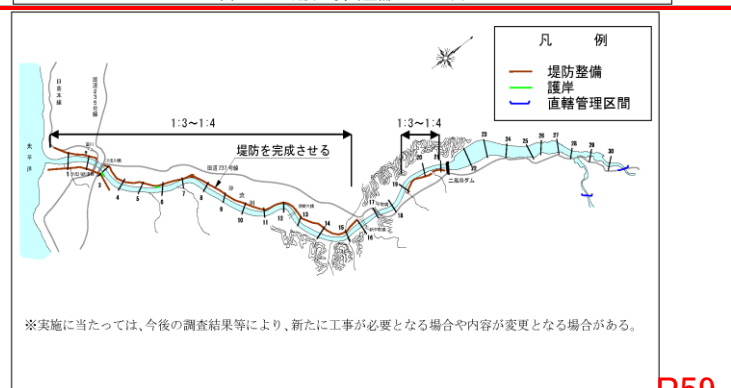
図 2-1-10 堤防整備箇所図
