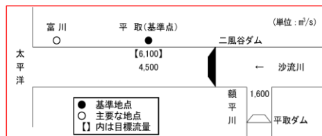
図 1-11 前河川整備計画（平成19年（2007年）3月）における河道への配分流量
