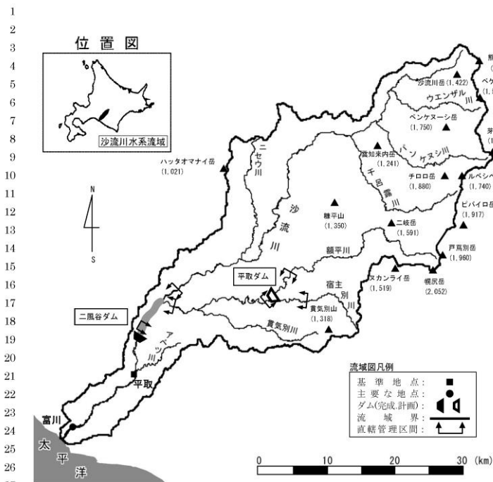
図 2-1-2 二風谷ダム及び平取ダム位置図
