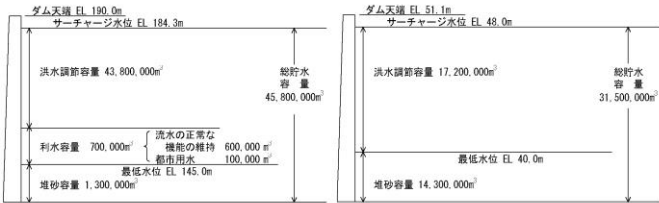
図 2-1-5 平取ダム貯水池容量配分図
