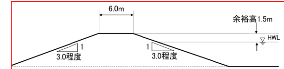
図 2-1 堤防整備の標準断面図（沙流川）
