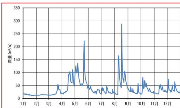
図 1-17 日平均流量の年変化（沙流川 基準地点平取、令和元年（2019年））
