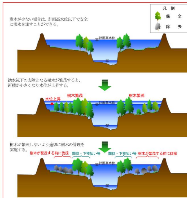
図 2-9 河道内樹木の管理イメージ図
