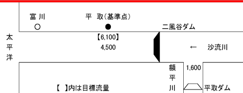
図 2-1-1 洪水調節計画流量配分図 [単位： \text{m}^3/\text{s} ]
