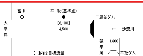
図 2-1-1 洪水調節計画流量配分図 [単位: \text{m}^3/\text{s} ]
