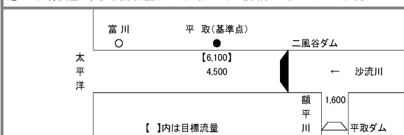
図 2-1-1 洪水調節計画流量配分図 [単位: m 3 /s]
