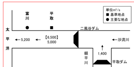
図 1-26 主要な地点における河道への配分流量 (単位: \text{m}^3/\text{s} )
