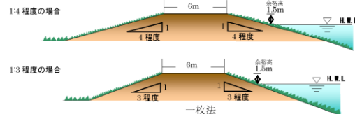
図 2-1-9 堤防の質的整備イメージ図
