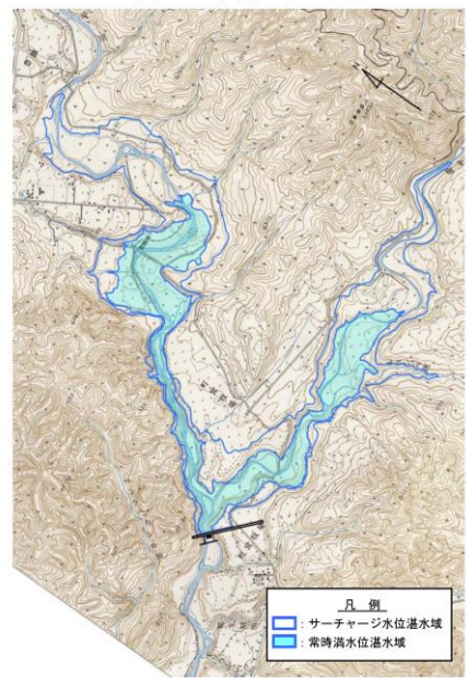
図 2-1-4 平取ダム貯水池平面図
