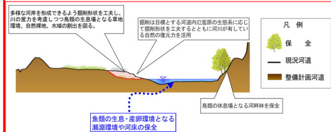
図 2-6 河畔林の保全、河岸の多様性の保全・創出イメージ図
