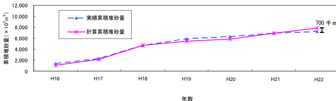
図 4.1-6 堆砂量の計算値と実測値の比較
