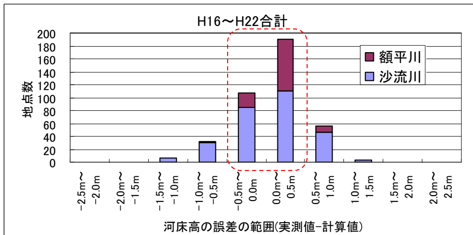
図 4.1-8 河床高の誤差の範囲(実測値-計算値)
