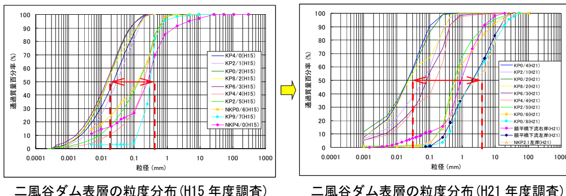
図 4.1-4 二風谷ダム表層の粒度の変化
