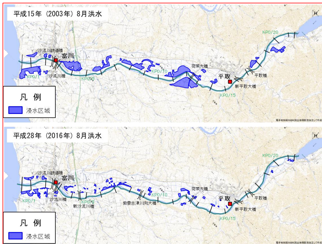
図 1-13 実績浸水図
