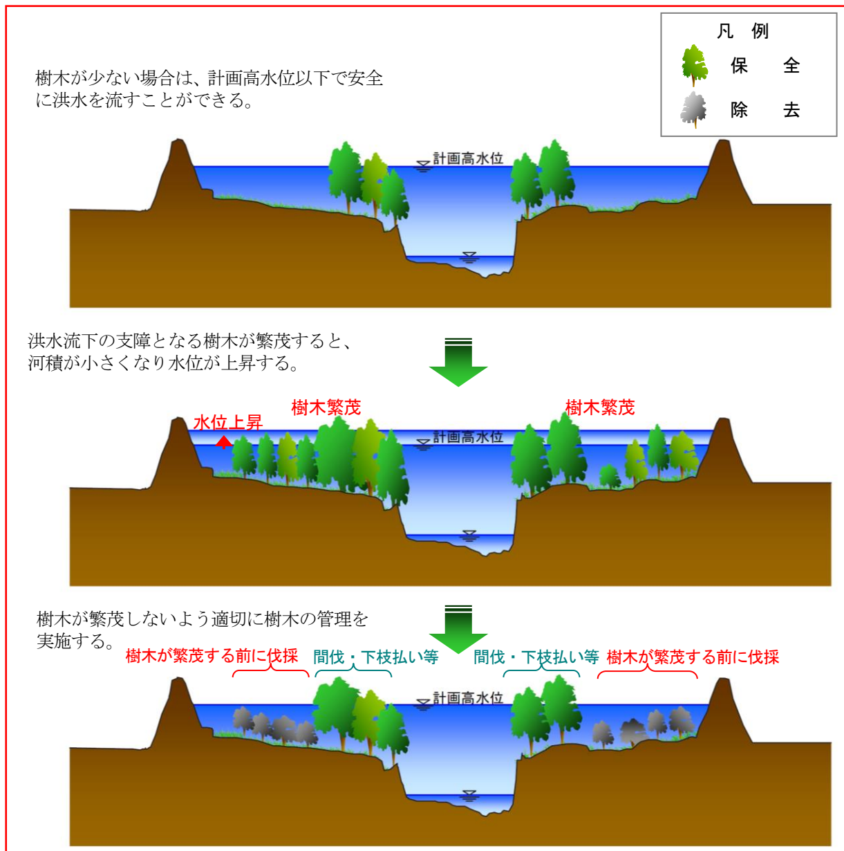
34 図 2-9 河道内樹木の管理イメージ図
