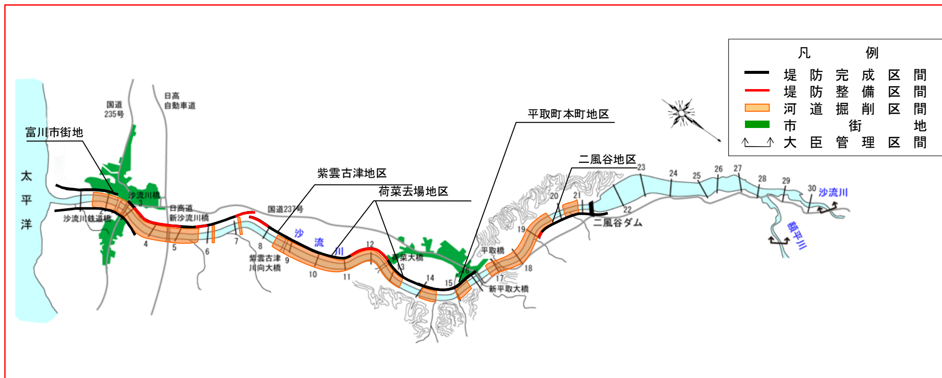
沙流川 整備計画平面図
