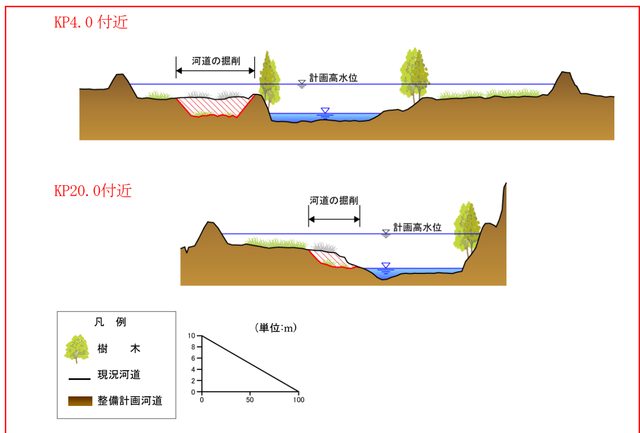
図 2-2 河道の掘削のイメージ図
