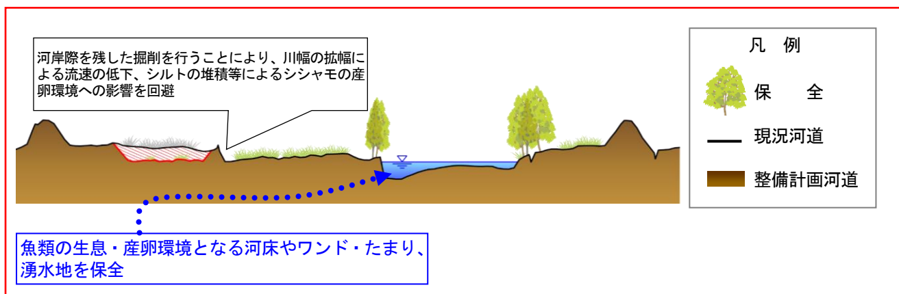
図 2-7 河道掘削のイメージ図
