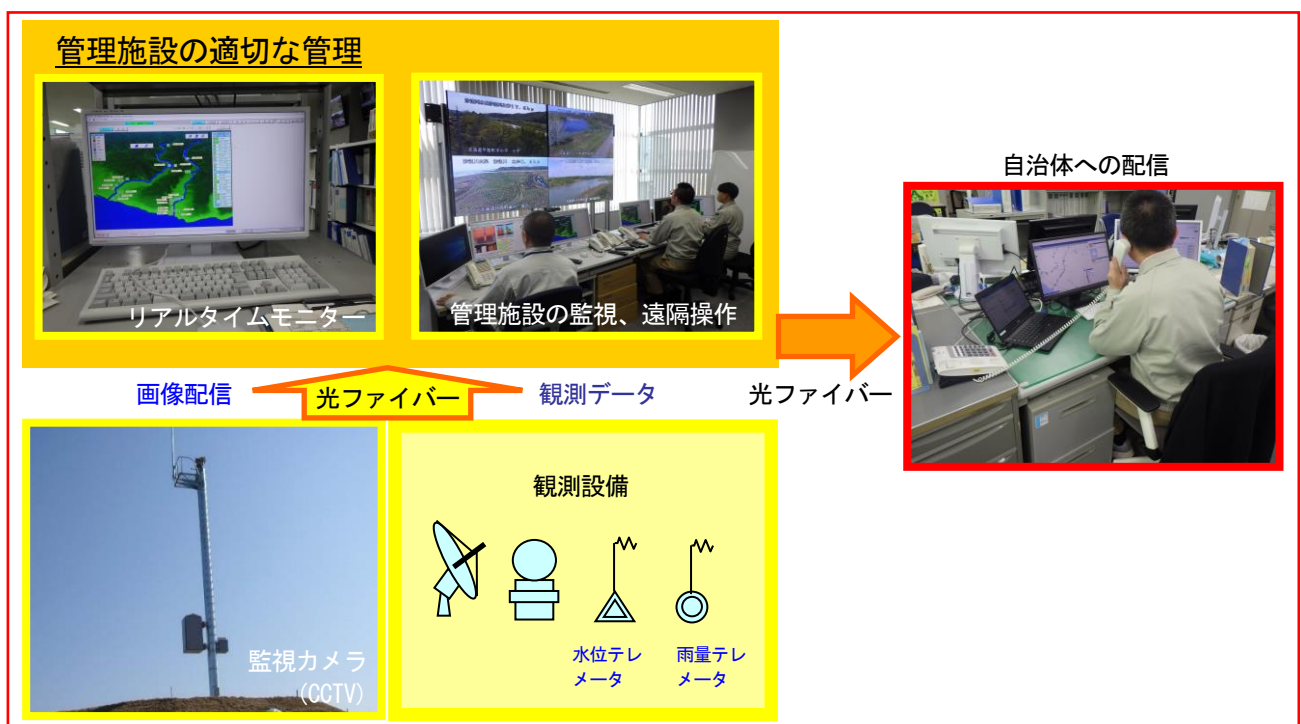
図 2-5 光ファイバー網による河川情報の収集・伝達のイメージ図
