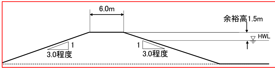
図 2-1 堤防整備の標準断面図（沙流川）
