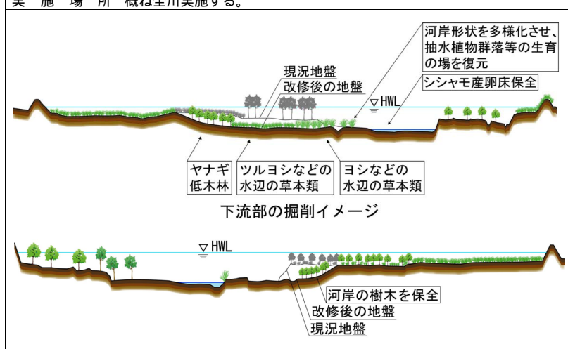
図 2-1-7 流下能力不足により対策が必要な断面横断面
