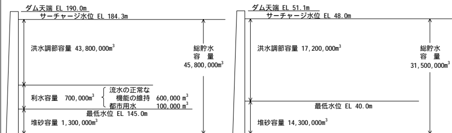
図 2-1-5 平取ダム貯水池容量配分図
