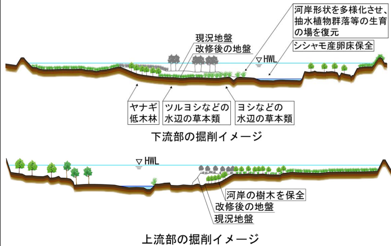
図 2-1-7 流下能力不足により対策が必要な断面横断面 (S = 1:5,000)
