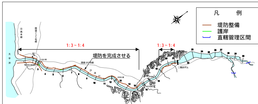
一枚法 図 2-1-9 堤防の質的整備イメージ図
