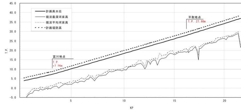
沙流川 計画縦断面図
