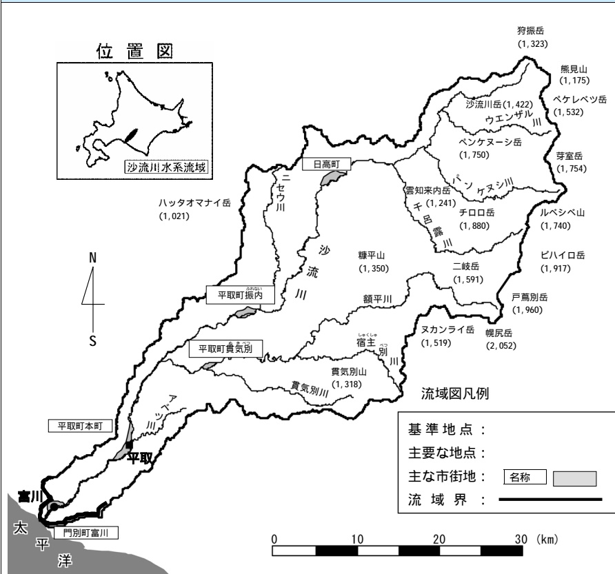
図 1-1-1 沙流川水系 概要図
