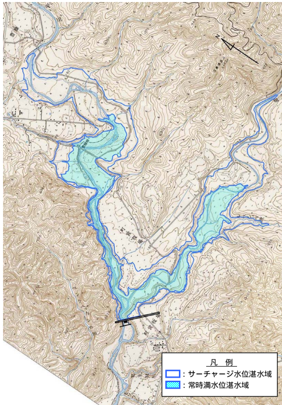
図 2-1-4 平取ダム貯水池平面図
