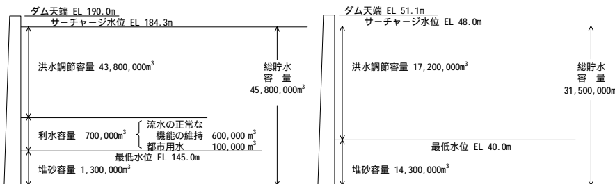
図 2-1-5 平取ダム貯水池容量配分図
