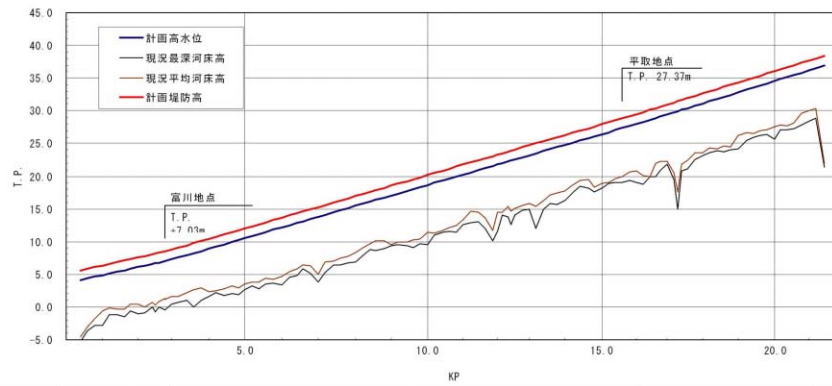
沙流川 計画縦断面図
