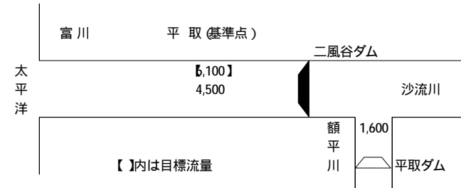
図 2-1-1 洪水調節計画流量配分図 [単位: m³/s]
