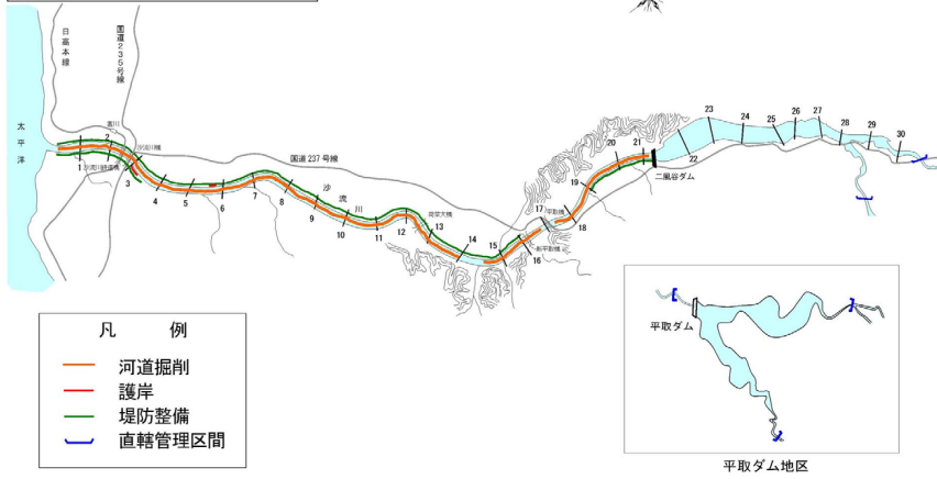
沙流川 河川整備計画平面図
