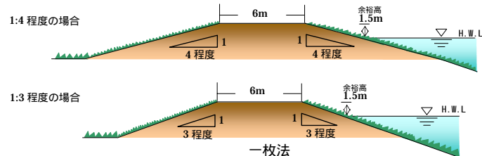
図 2-1-9 堤防の質的整備イメージ図
