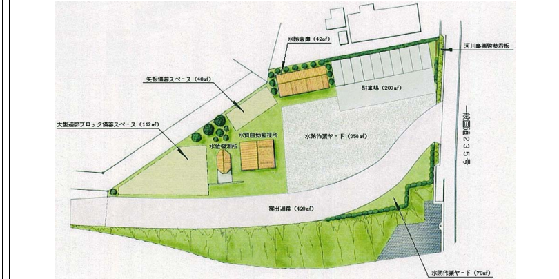
図 2-1-15 富川地区防災拠点施設配置図
