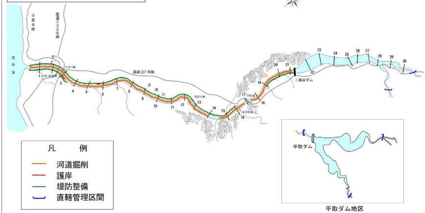
沙流川 河川整備計画平面図
