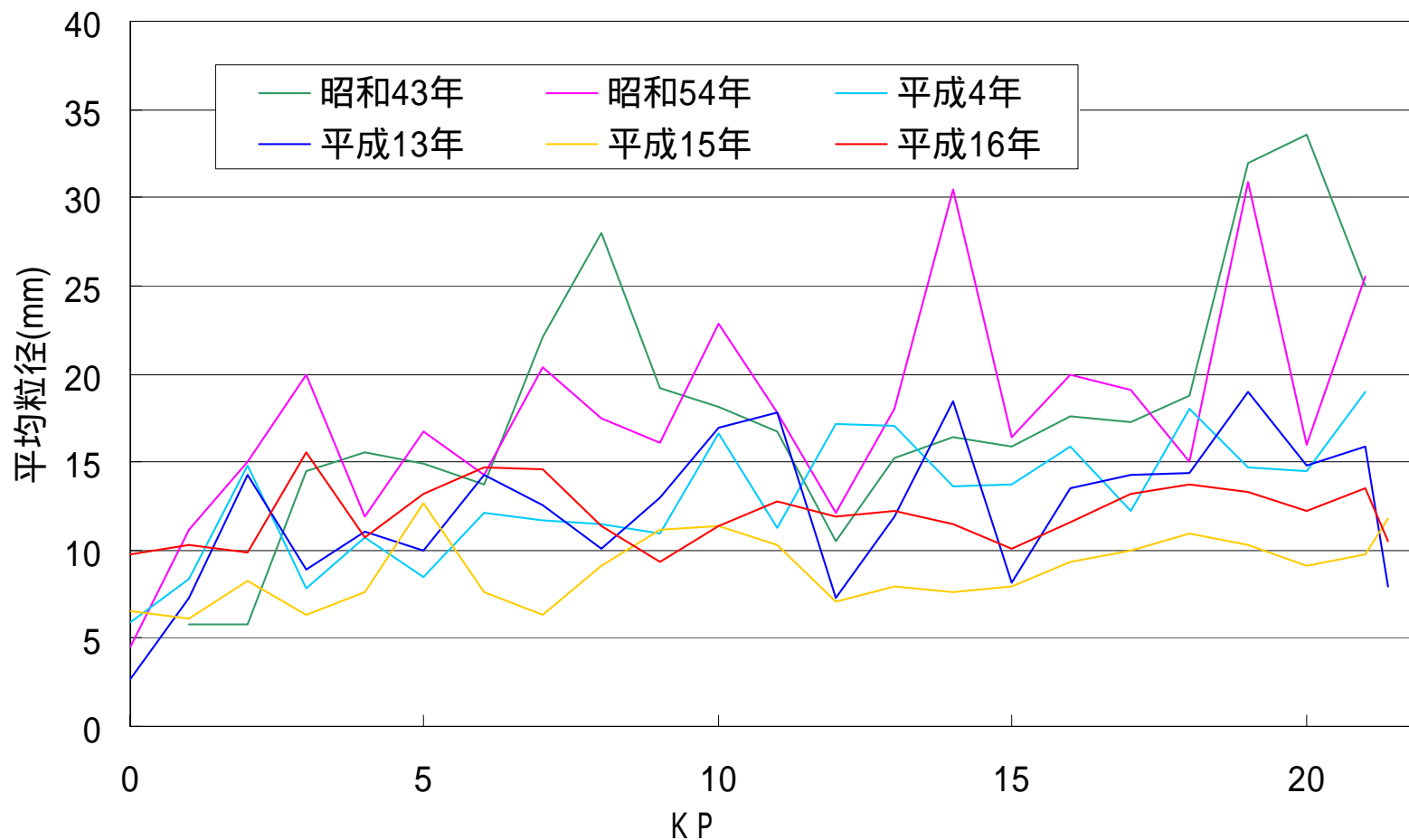
河床材料の平均粒径の変遷
