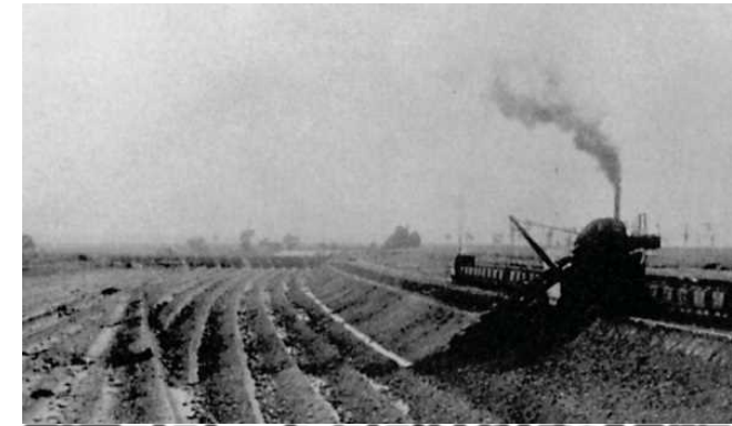
掘削機工キスカベーターによる統内新水路の作業状況
