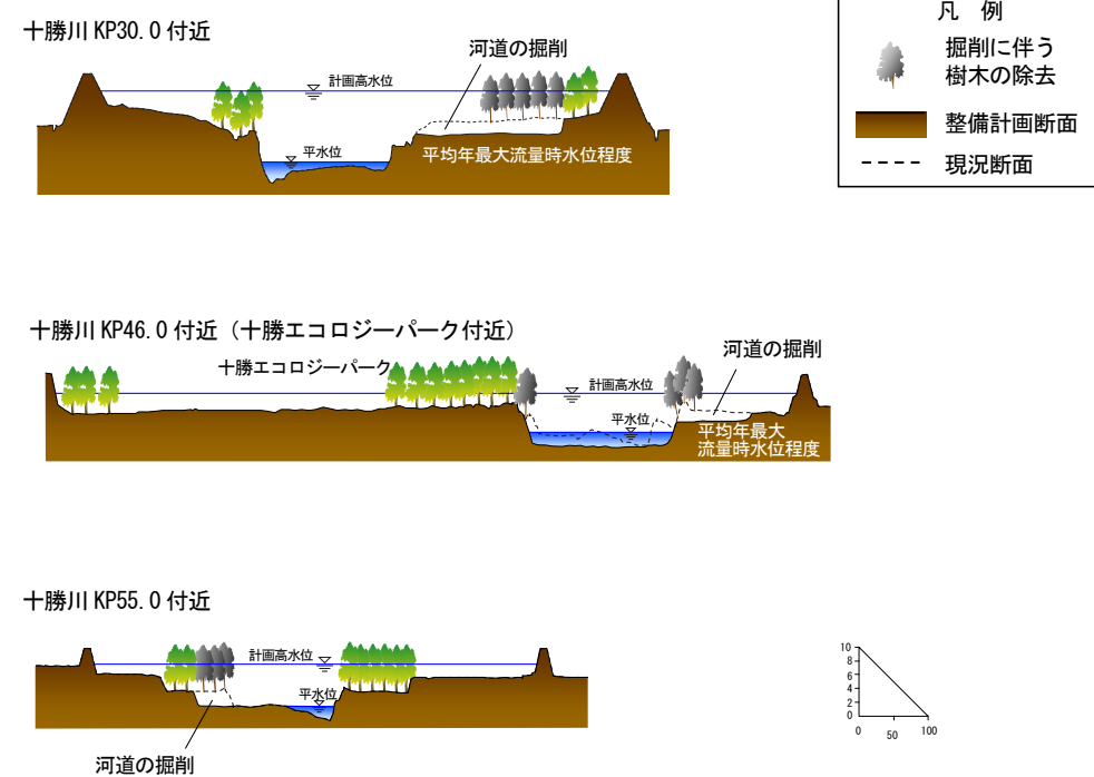
図 2-5 河道の掘削のイメージ図（十勝川）
