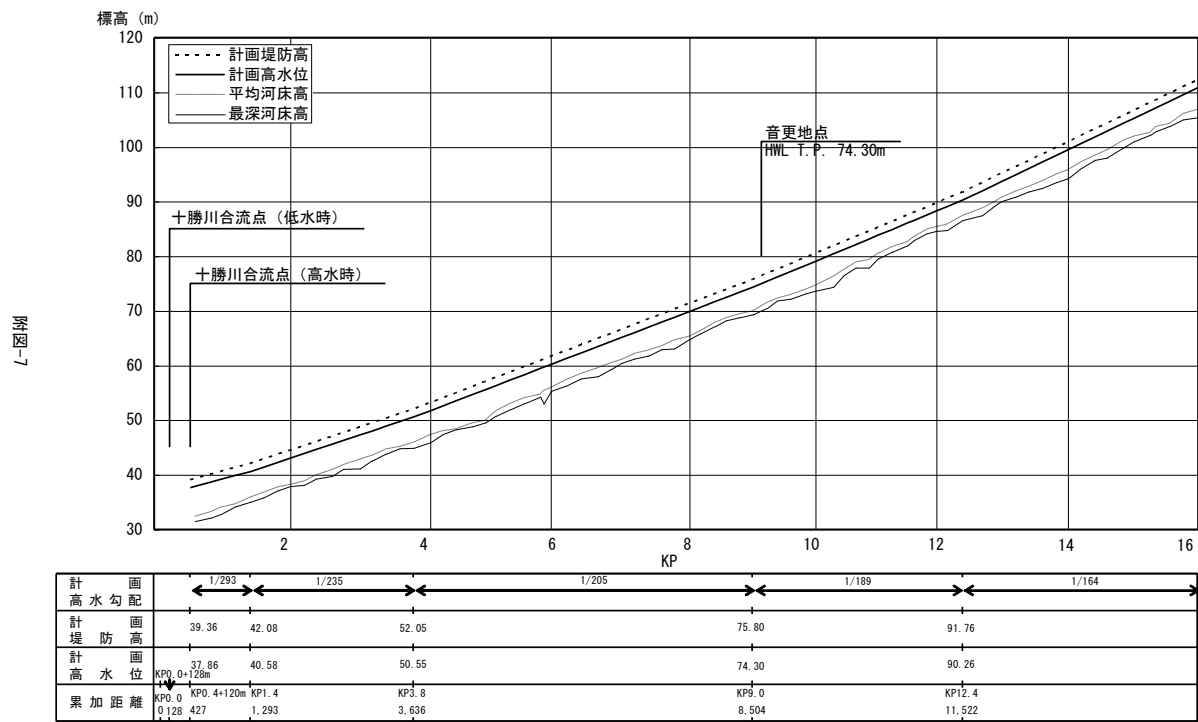
音更川計画縦断面図（1 / 2）
