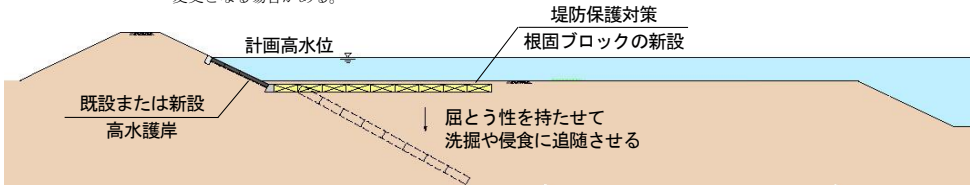
図 2-3 堤防の保護対策のイメージ図
