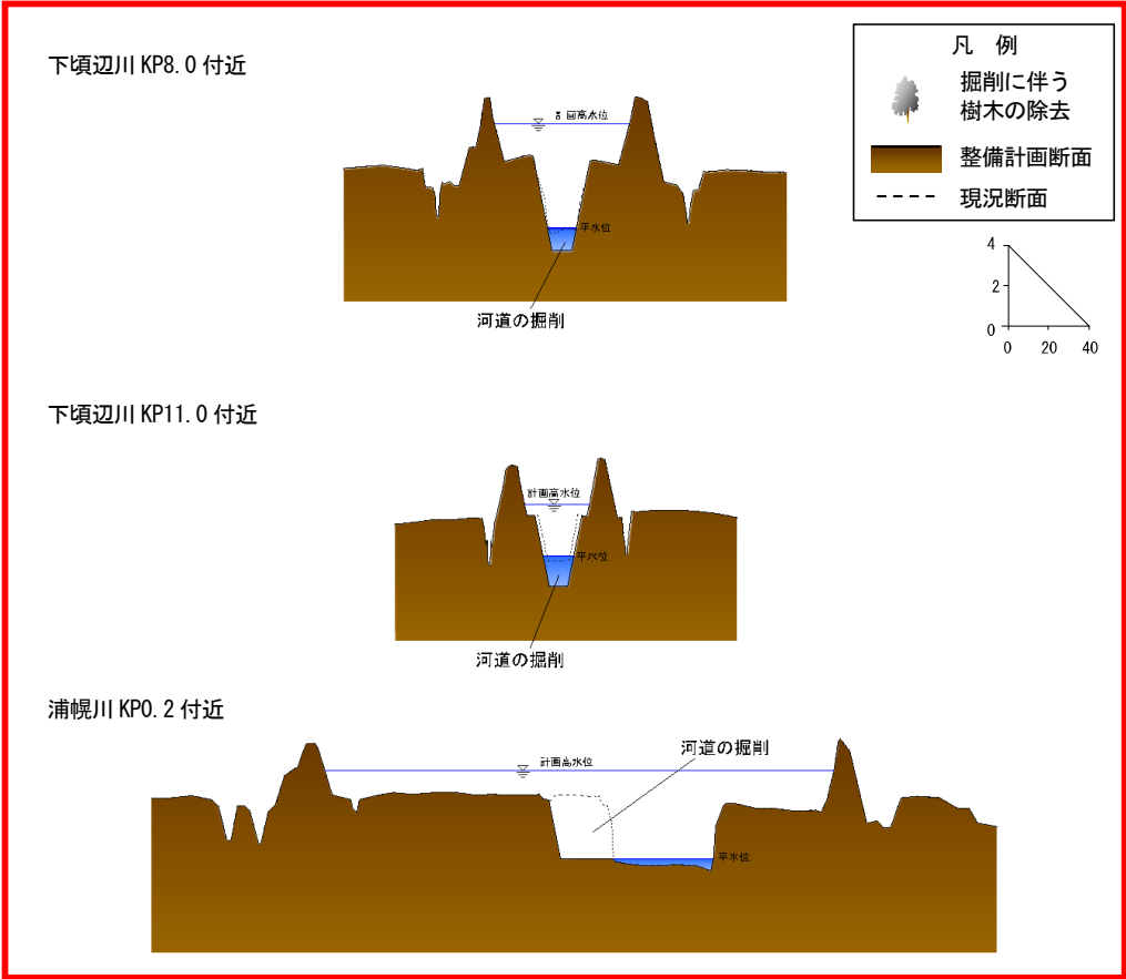
図 2-7(2) 河道の掘削のイメージ図（下頃辺川、浦幌川）
