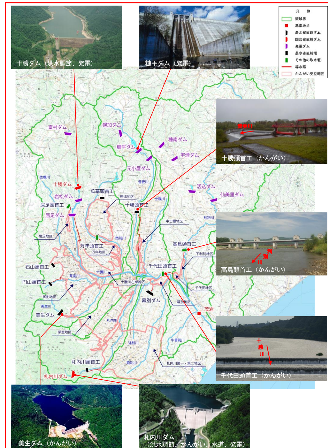
図 1-23 十勝川流域における主な水利用施設
