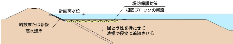
図 2-2 堤防の保護対策のイメージ図
