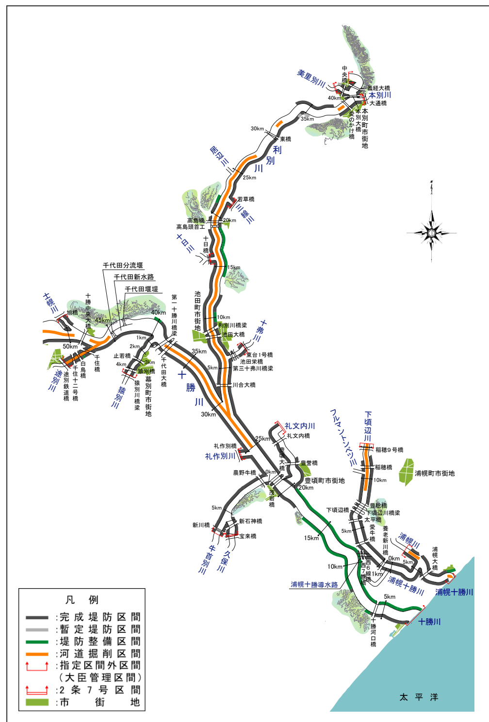
図 2-7(2) 堤防の整備、河道の掘削等を実施する区間（十勝川、利別川、浦幌十勝川・下頃辺川）
