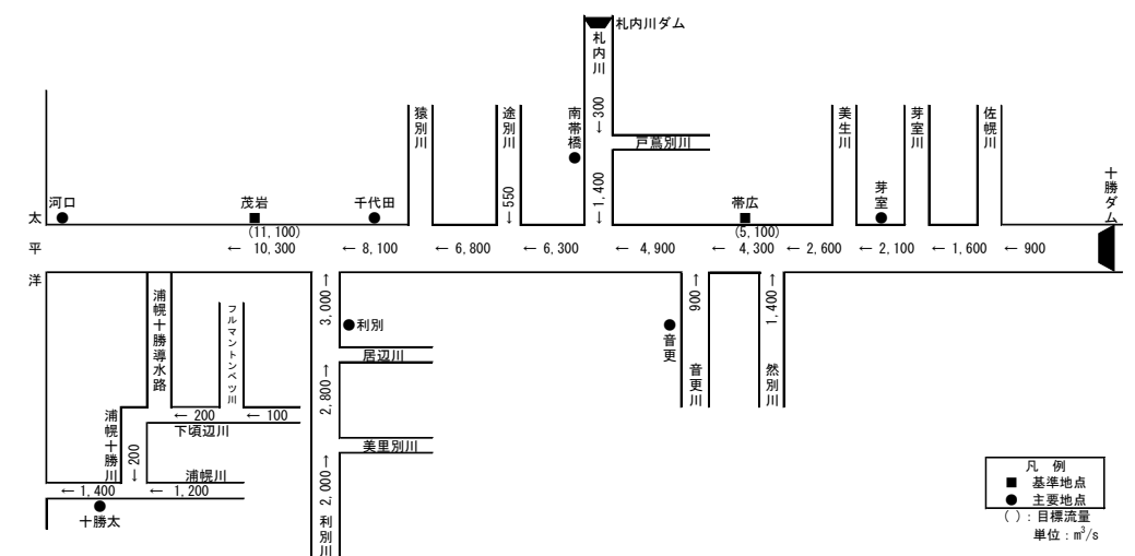
図 1-15 前河川整備計画（平成 25 年(2013 年)6 月）における主要な地点の河道への配分流量
