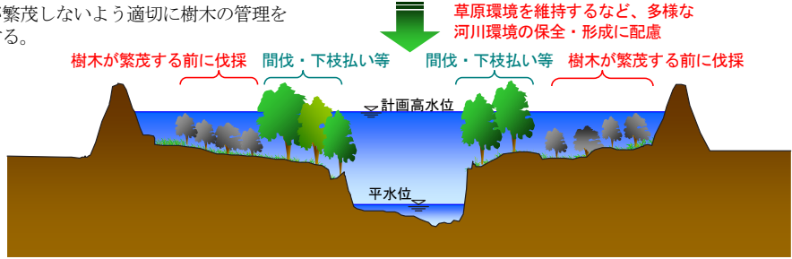
図 2-18 河道内樹木の管理イメージ図
