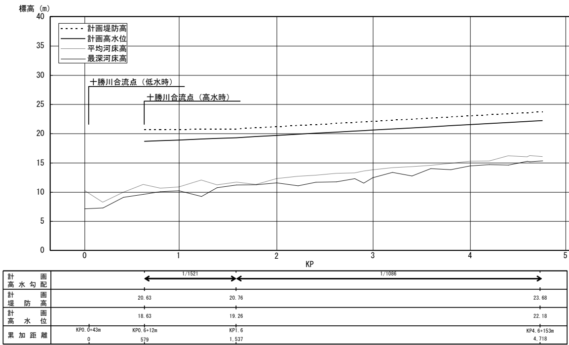
猿別川計画縦断面図
