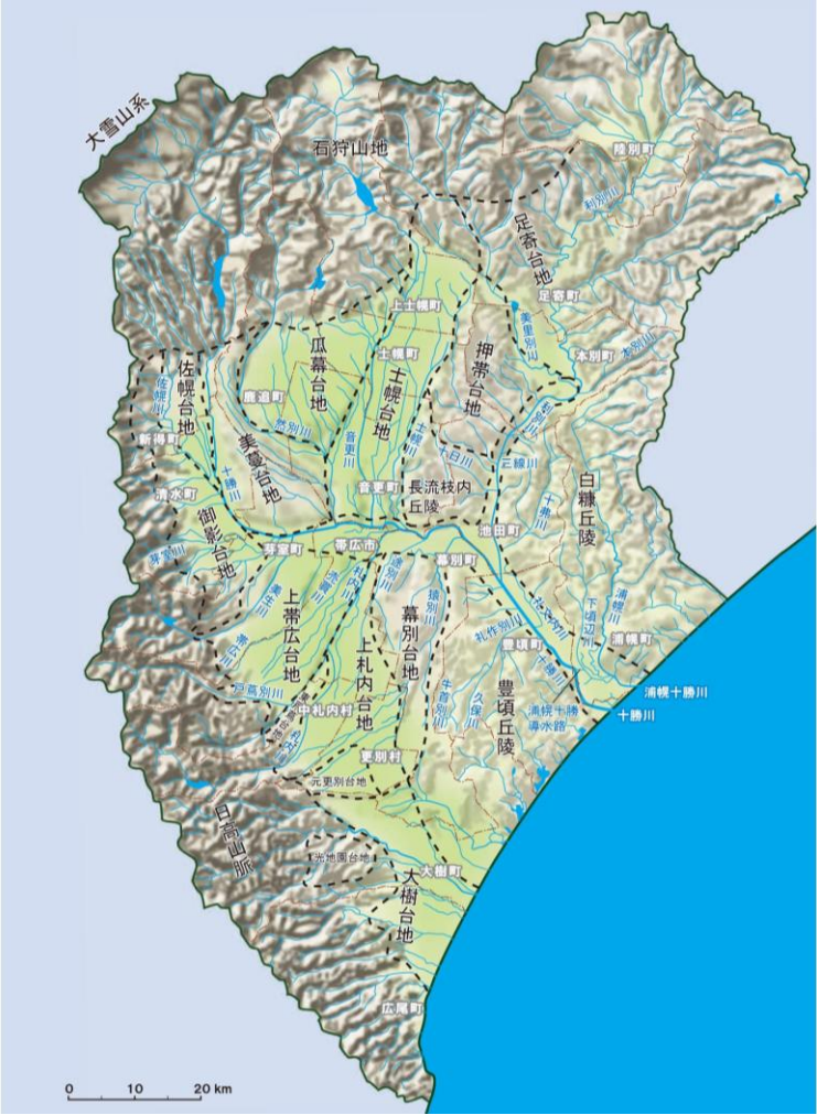
図 1-2 十勝川流域の地形
