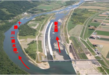
千代田新水路
