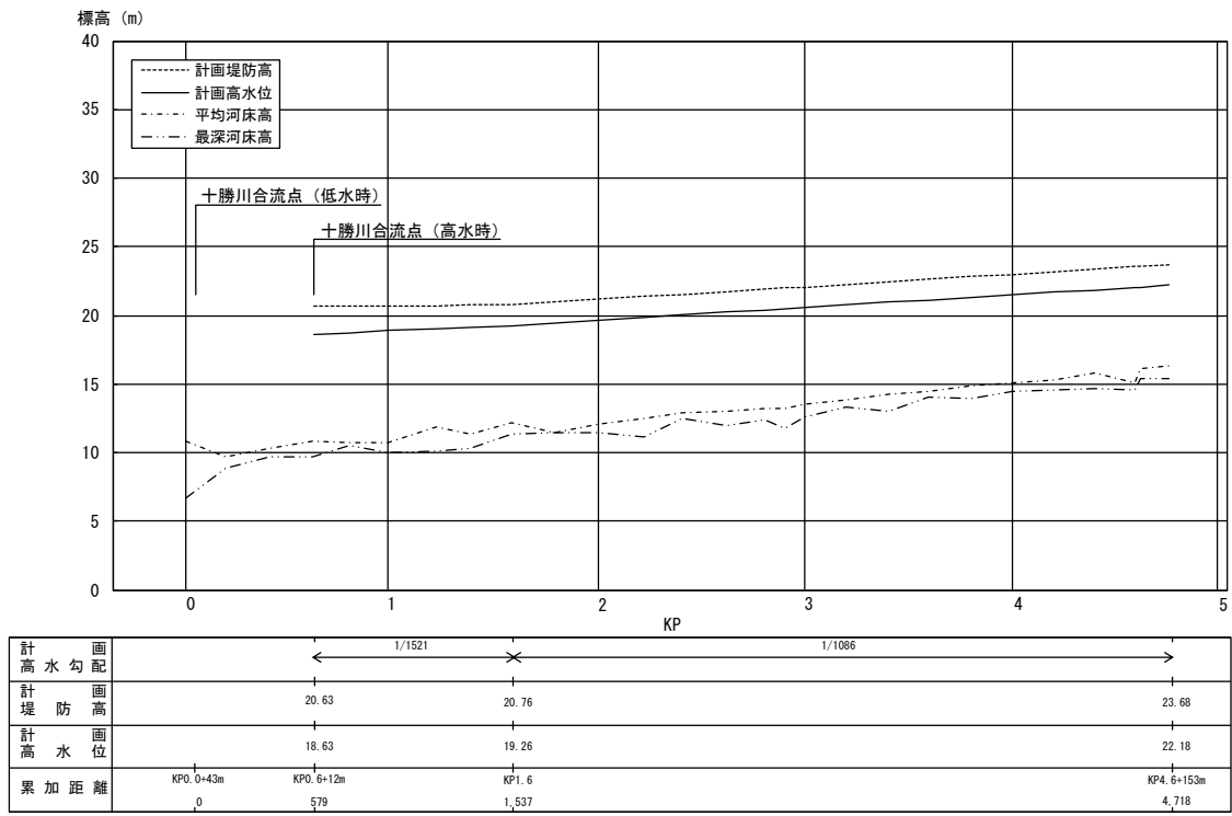
猿別川計画縦断面図
