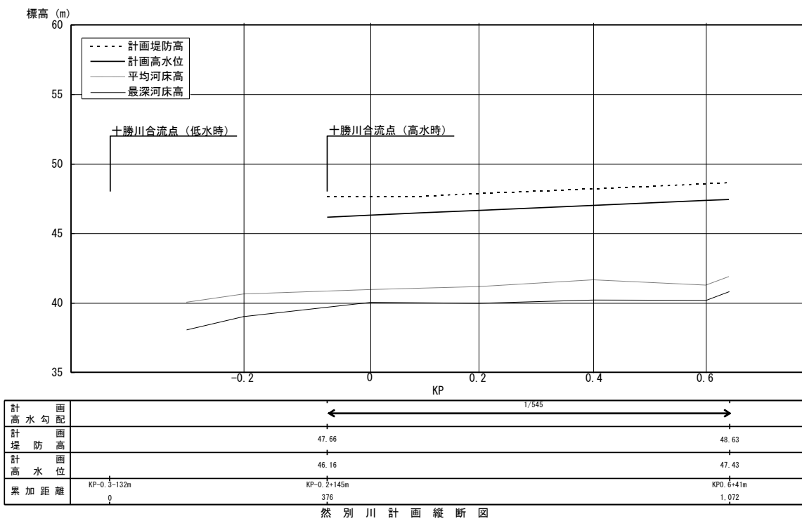
然別川計画縦断面図
