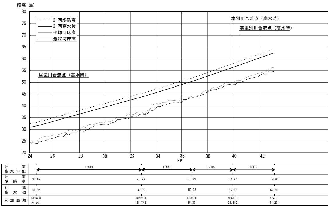
利別川計画縦断面図（2 / 2）
