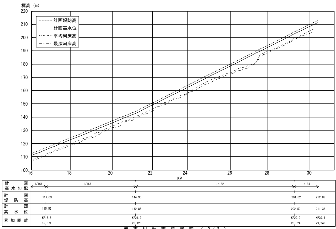
音更川計画縦断面図（2 / 2）
