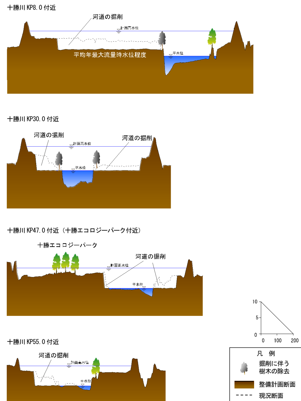
図 2-4(1) 河道の掘削のイメージ図（十勝川）
