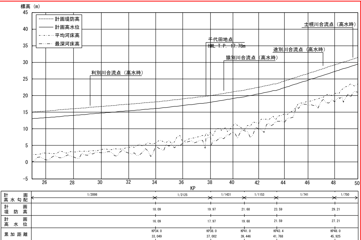
十勝川計画縦断面図（2 / 4）
