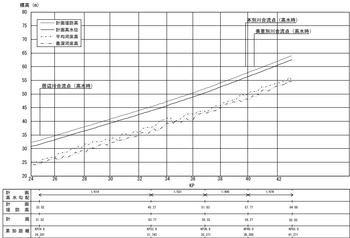
利別川計画縦断面図（2 / 2）
