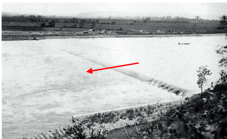
千代田堰堤全景(昭和 10 年)
