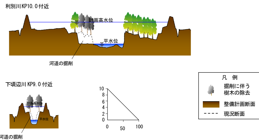
図 2-6 河道の掘削のイメージ図（利別川、浦幌十勝川・下頃辺川）
