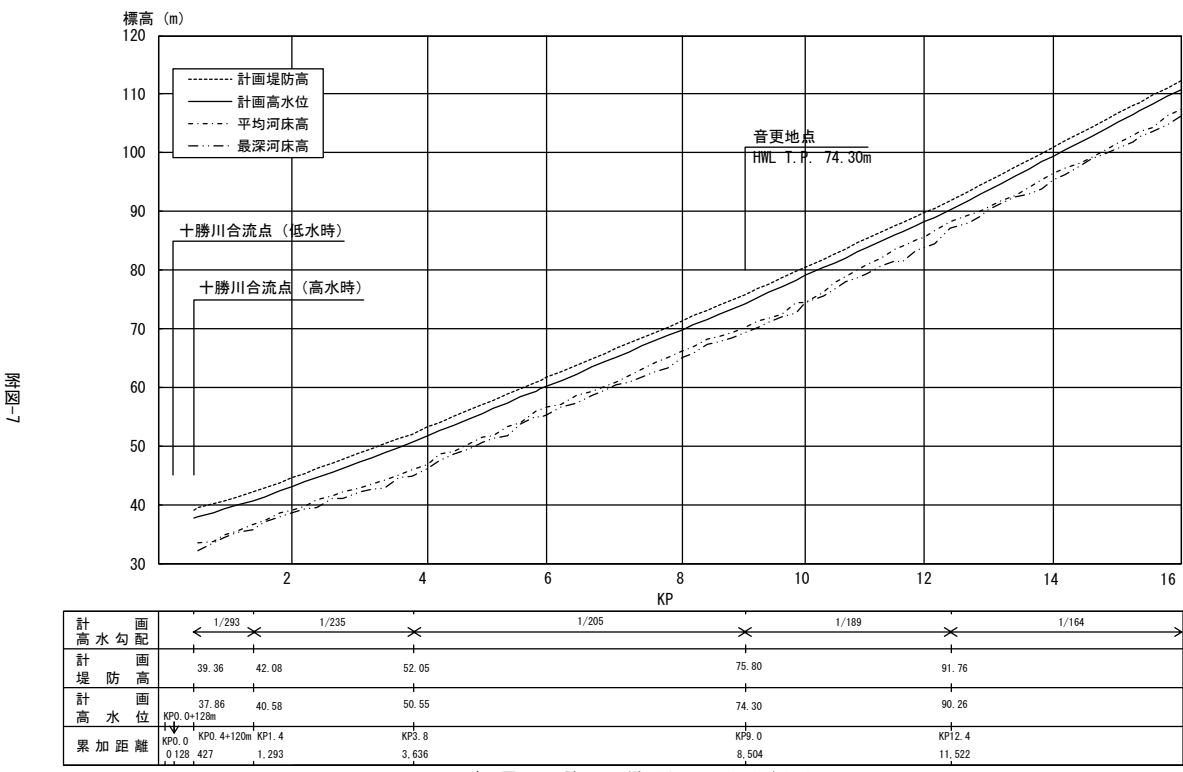
音更川計画縦断面図（1 / 2）
