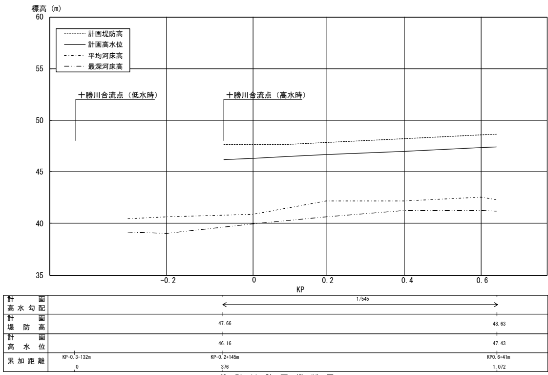
然別川計画縦断面図
