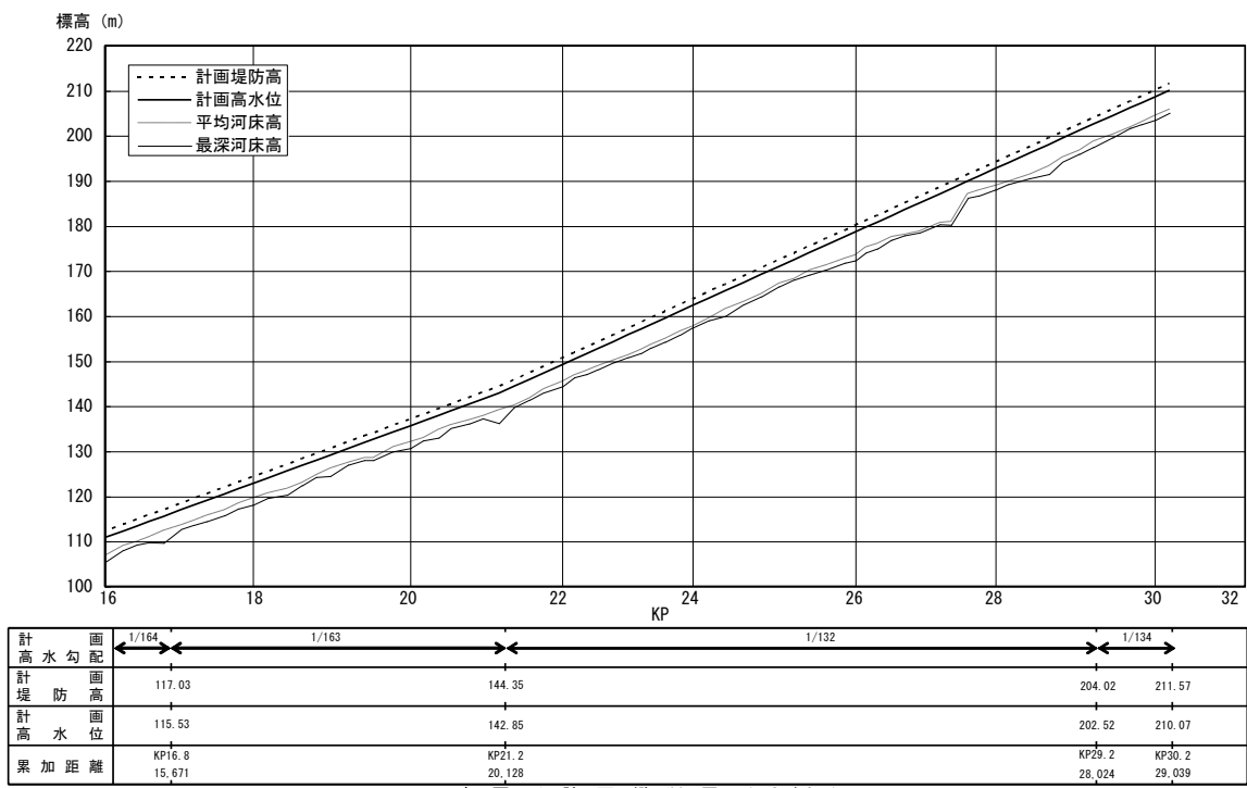
音更川計画縦断面図（2 / 2）
