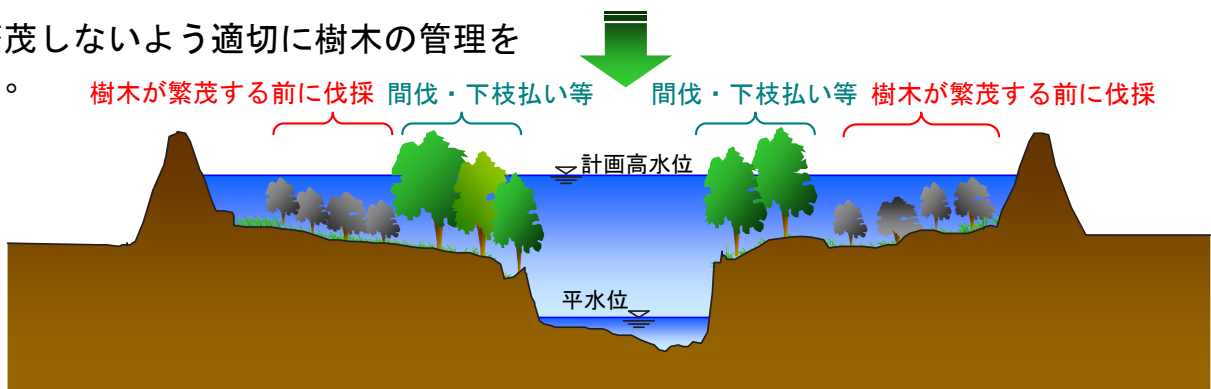
河道内樹木の管理イメージ図
