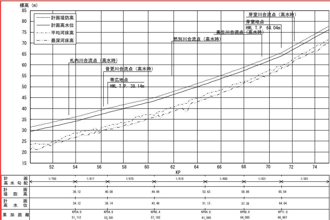
十勝川計画縦断面図（3 / 4）
