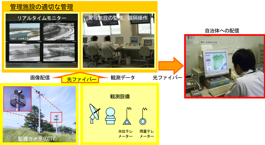
図 2-10 光ファイバー網による河川情報の収集・伝達のイメージ図
