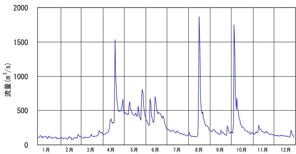
図 1-18 日平均流量の年変化（十勝川 茂岩地点 平成 18 年）
