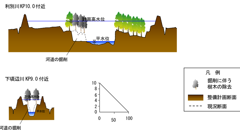
図 2-4 河道の掘削のイメージ図（利別川、浦幌十勝川・下頃辺川）
