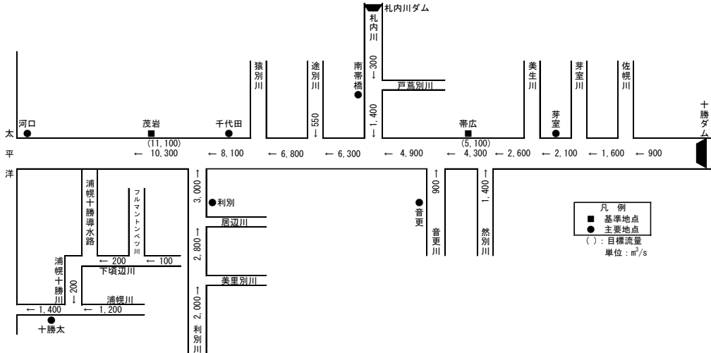
図 1-32 主要な地点における河道への配分流量
