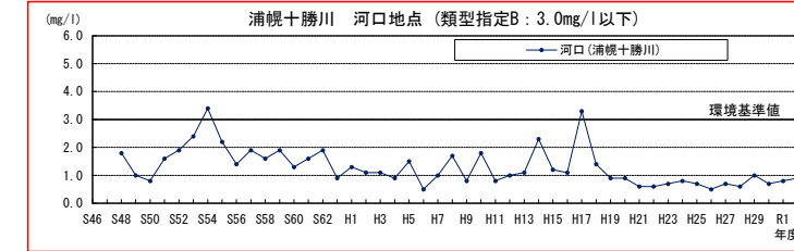
図 1-29 浦幌十勝川・下頃辺川における水質（BOD75%値）の経年変化
