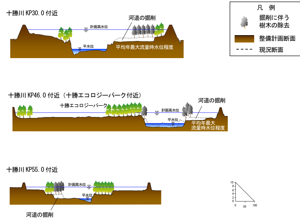
図 2-3 河道の掘削のイメージ図（十勝川）
