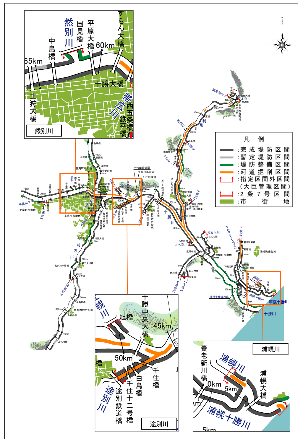
図 2-10 堤防の整備、河道の掘削等を実施する区間（中小支川）
