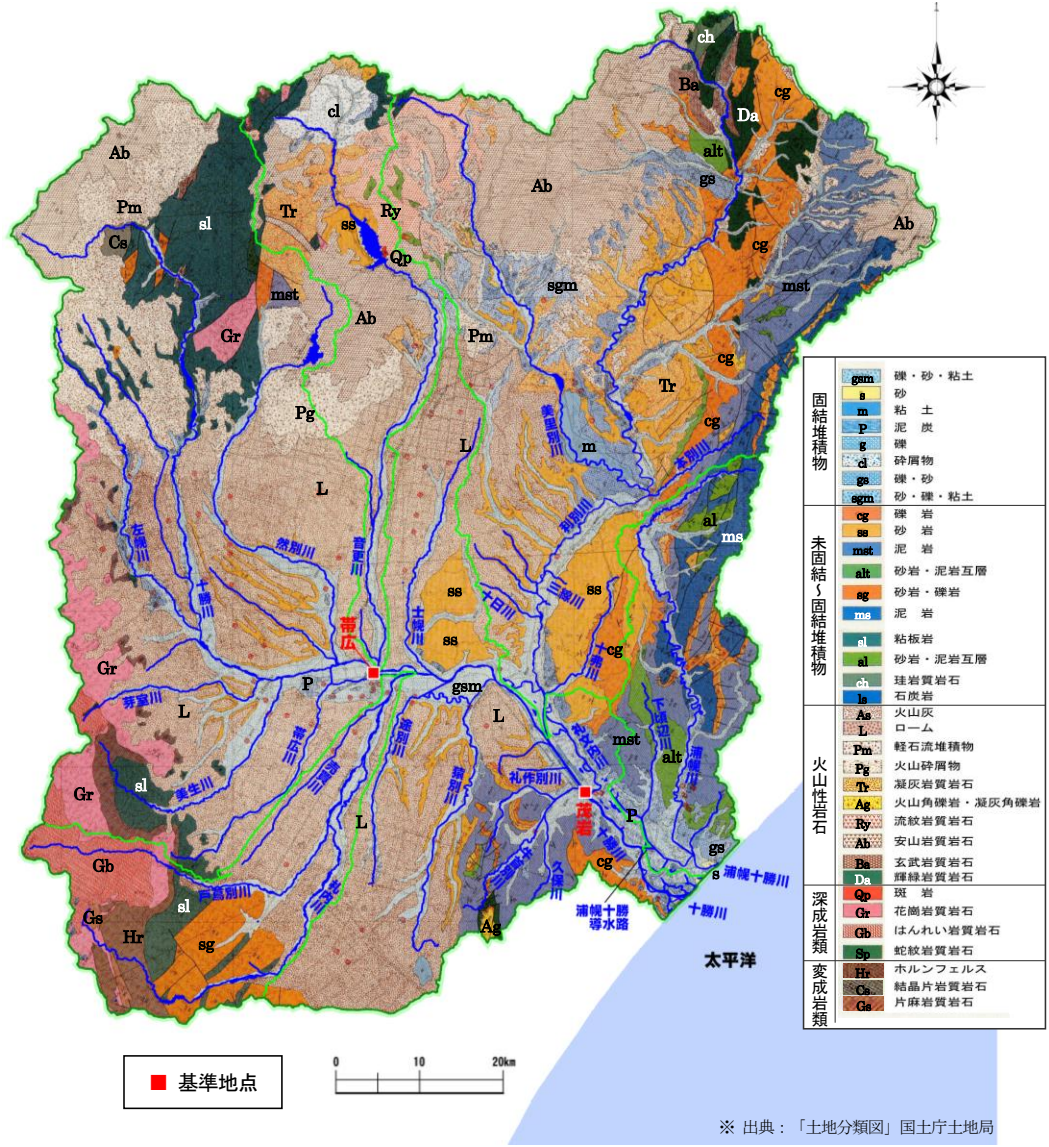
図 1-3 表層地質図
