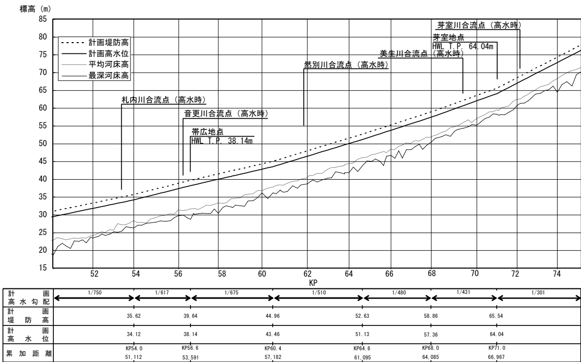
十勝川計画縦断面図（3 / 4）
