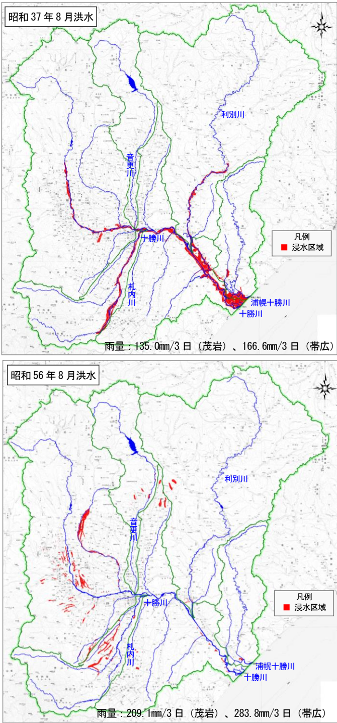
図 1-15(1) 主要洪水の浸水実績図
