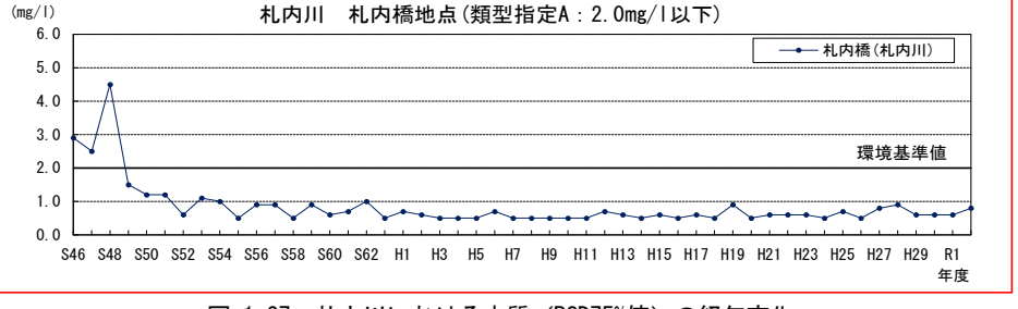
図 1-27 札内川における水質（BOD75%値）の経年変化
