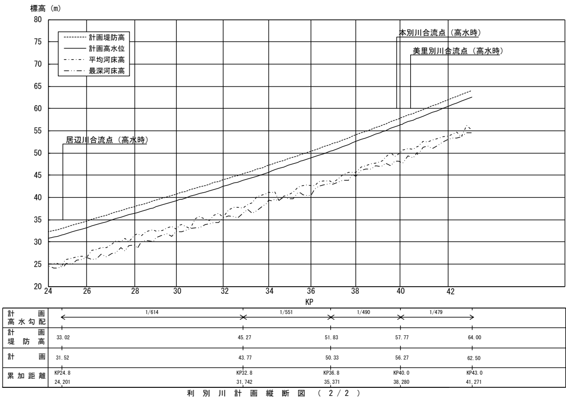
利別川計画縦断面図（2 / 2）
