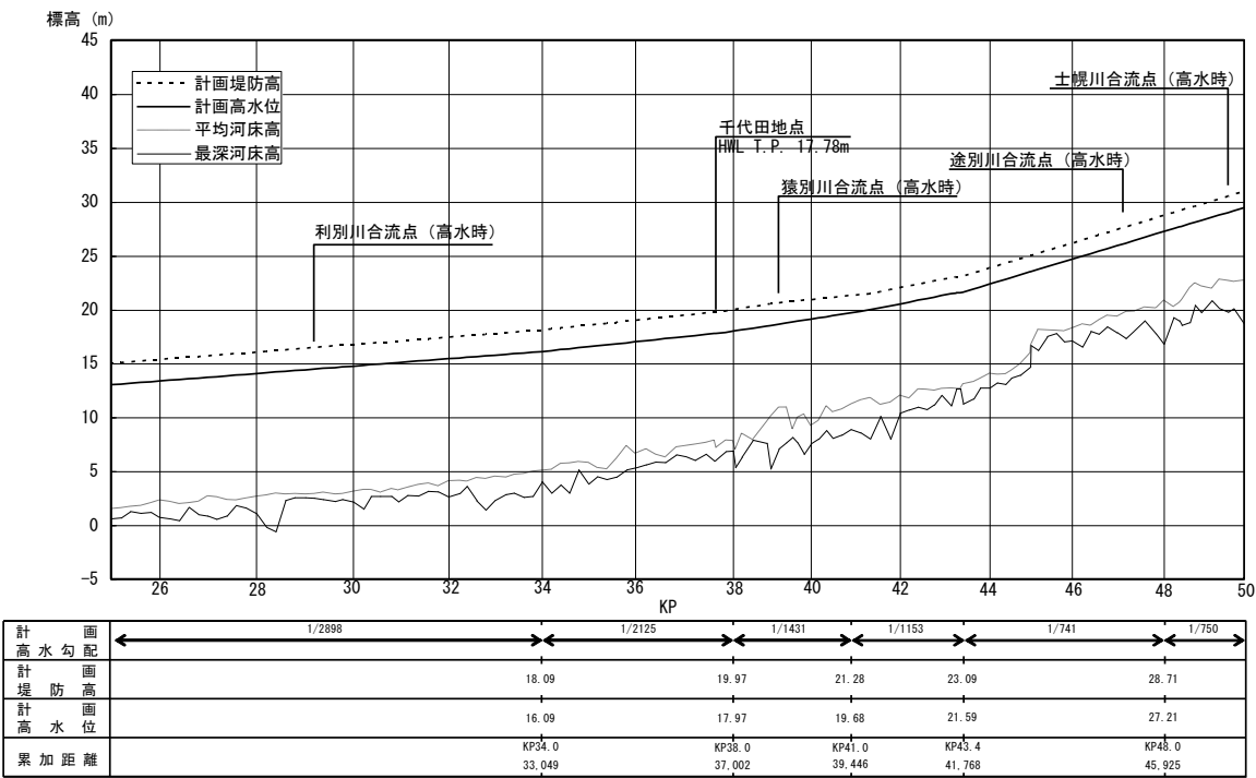
十勝川計画縦断面図（2 / 4）
