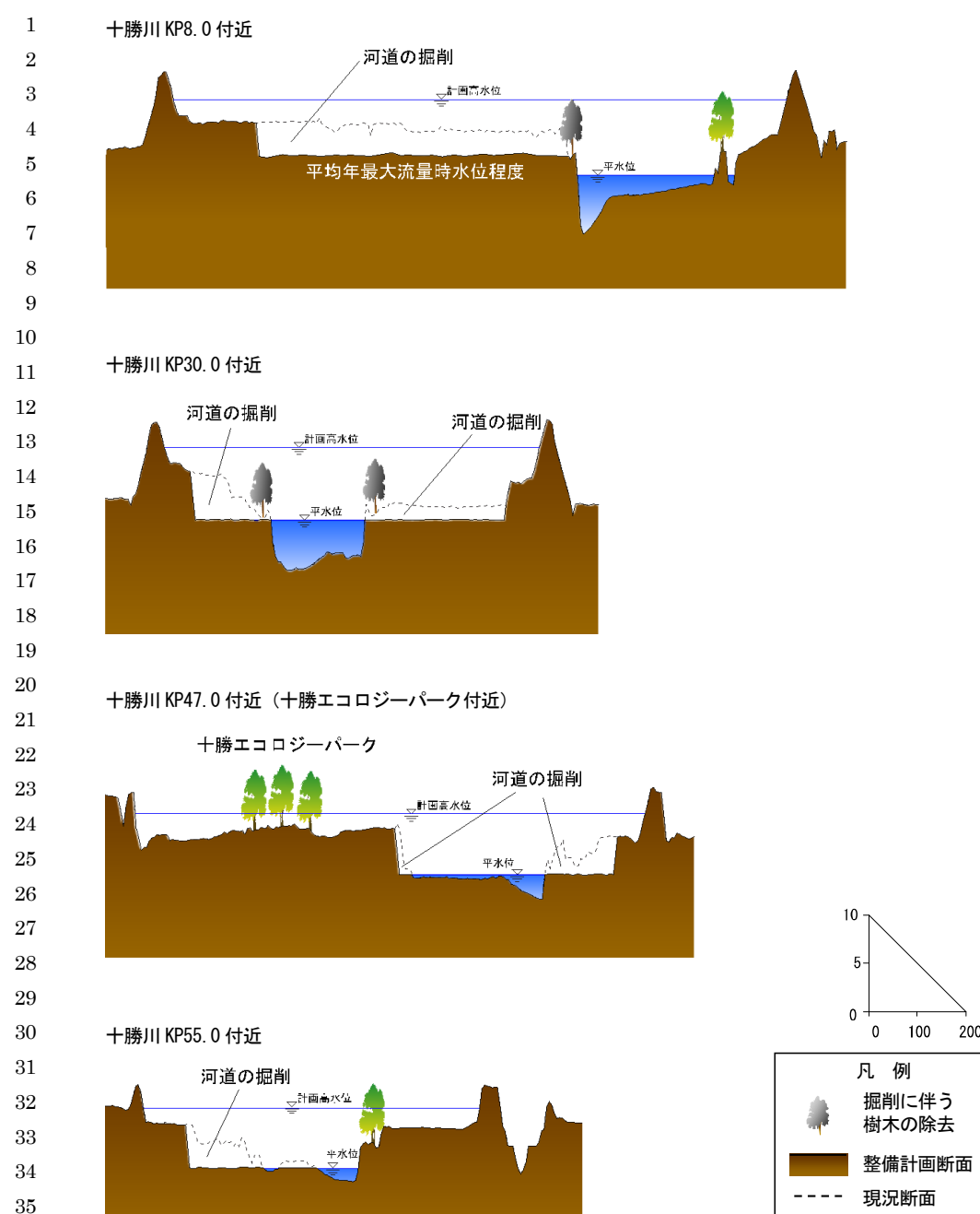
図 2-4(1) 河道の掘削のイメージ図（十勝川）
