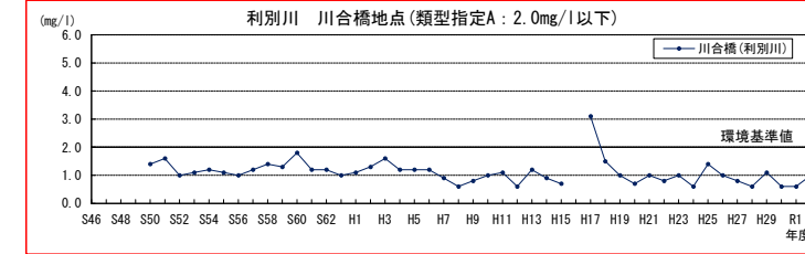
図 1-28 利別川における水質（BOD75%値）の経年変化
