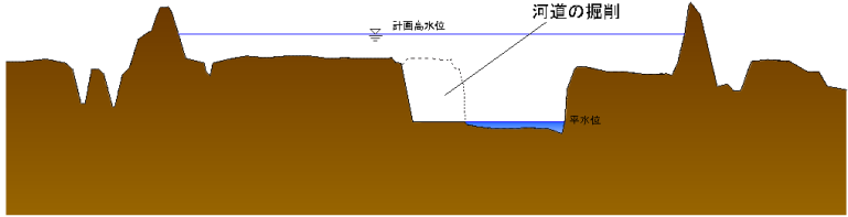
図 2-7(2) 河道の掘削のイメージ図（下頃辺川、浦幌川）
