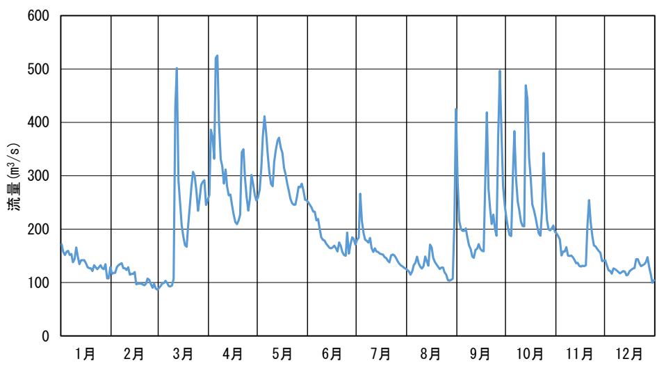
図 1-21 日平均流量の年変化（十勝川 茂岩地点 令和 2 年(2020 年)）
