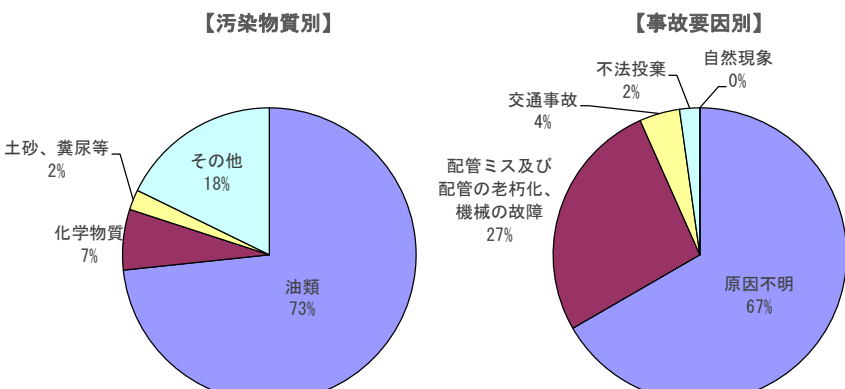
図 1-30 十勝川水系の水質事故原因（平成 24 年(2012 年)～令和 3 年(2021 年)）
