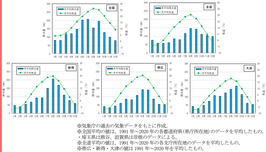
図 1-4 月別降水量、月別平均気温
