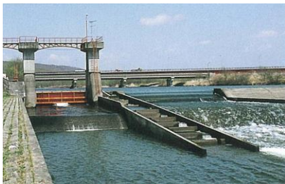
旧高島頭首工
