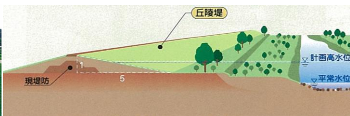
丘陵堤イメージ
