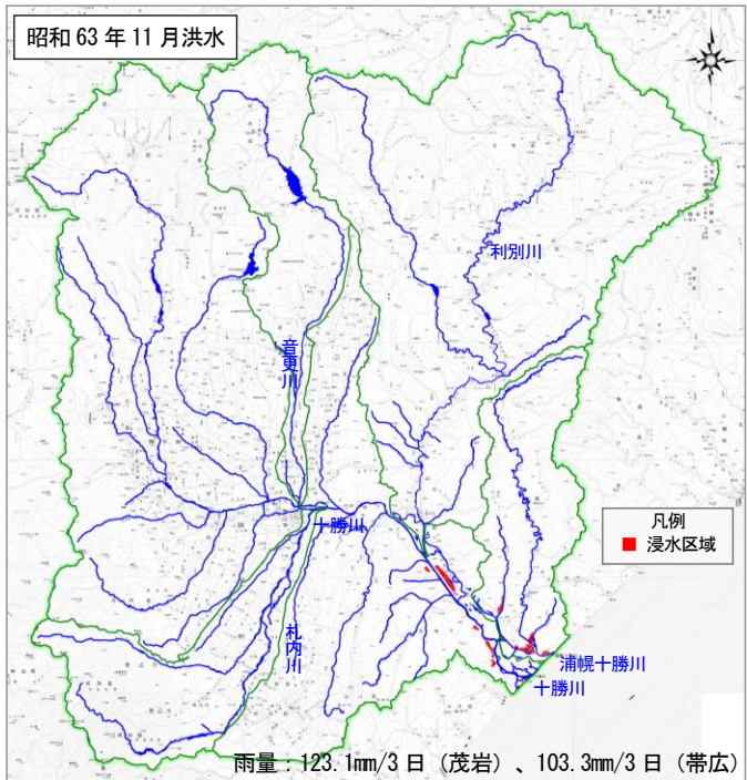
図 1-15(2) 主要洪水の浸水実績図
