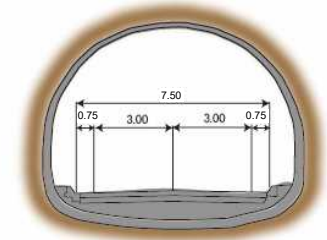
標準定規図
