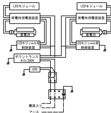
内部結線図
