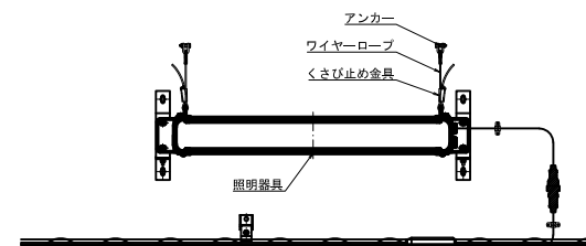
非常駐車帯照明
