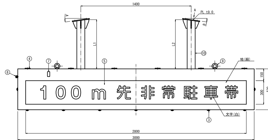
部材表 (非常駐車帯予告表示灯)
