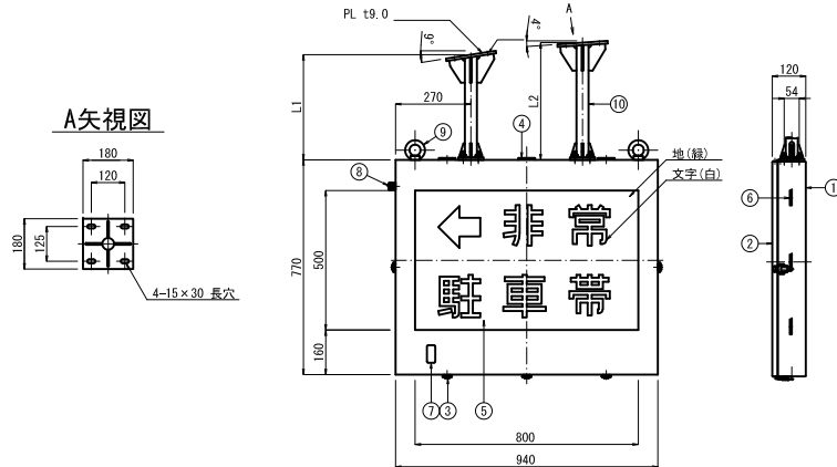
非常駐車帯表示灯
