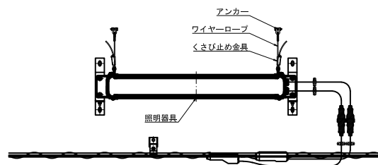
基本照明・入口照明
