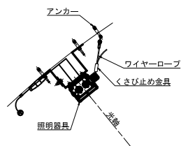
取付断面図
