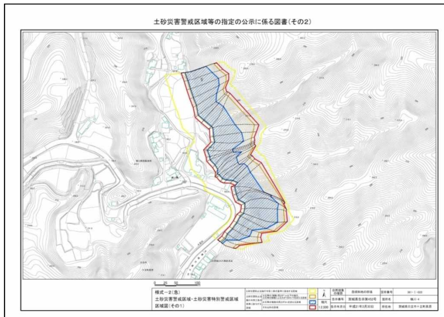
急傾斜地の崩壊に関する土砂災害警戒区域等の例
