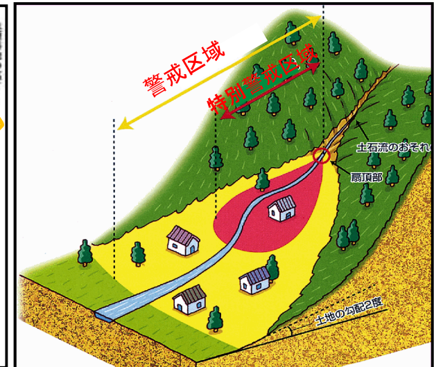
土石流に関する土砂災害警戒区域等の例
