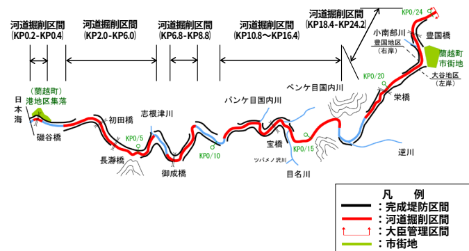
図 2-2 堤防の整備、河道の掘削を実施する区間
