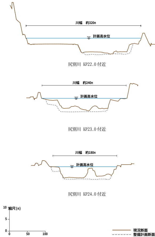
尻別川 横断面 (3/3)
