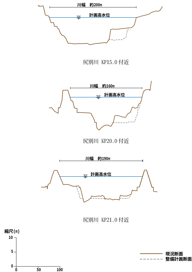
尻別川 横断面 (2/3)
