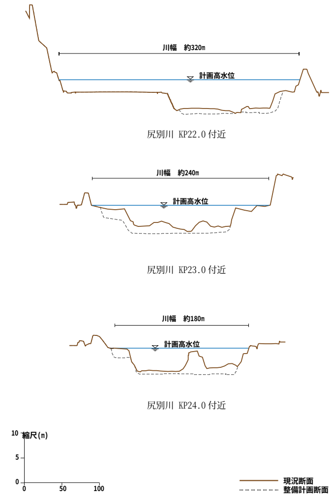
尻別川 横断面 (3/3)
