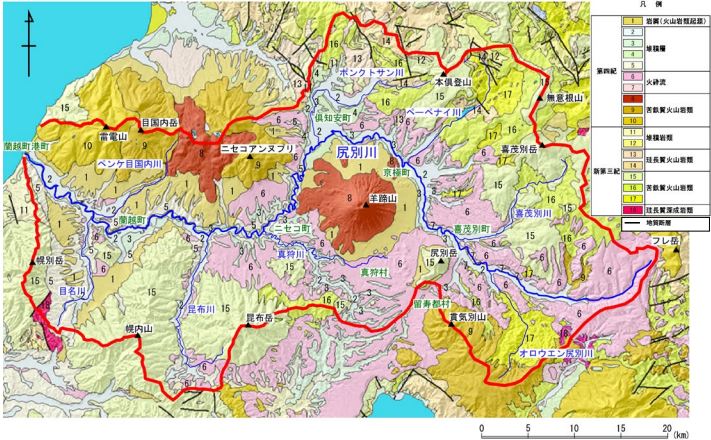
図 1-3 地質図
