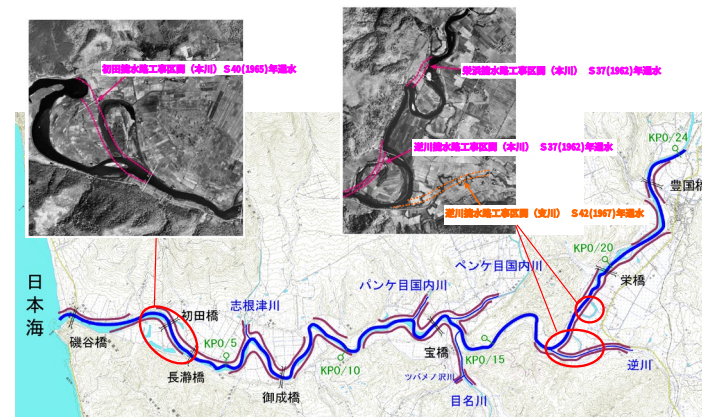
図 1-7 捷水路実施箇所
