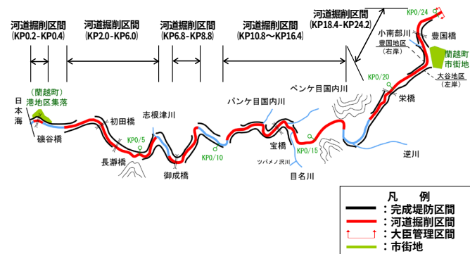
図 2-2 堤防の整備、河道の掘削を実施する区間
