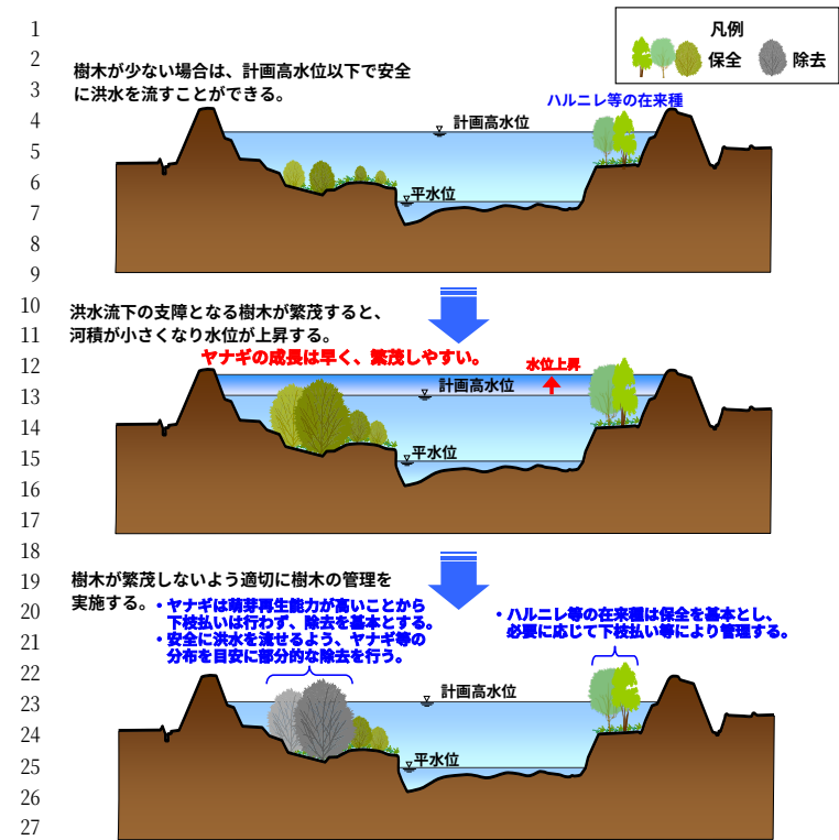
図 2-7 河道内樹木の管理イメージ図
