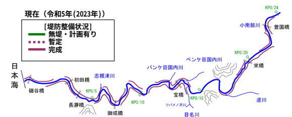
図 1-8 堤防整備の変遷(2)
