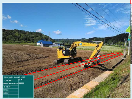
農業用排水路の施工状況
