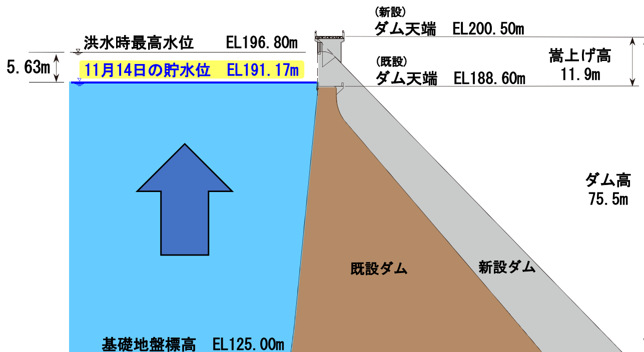
新桂沢ダム断面図
