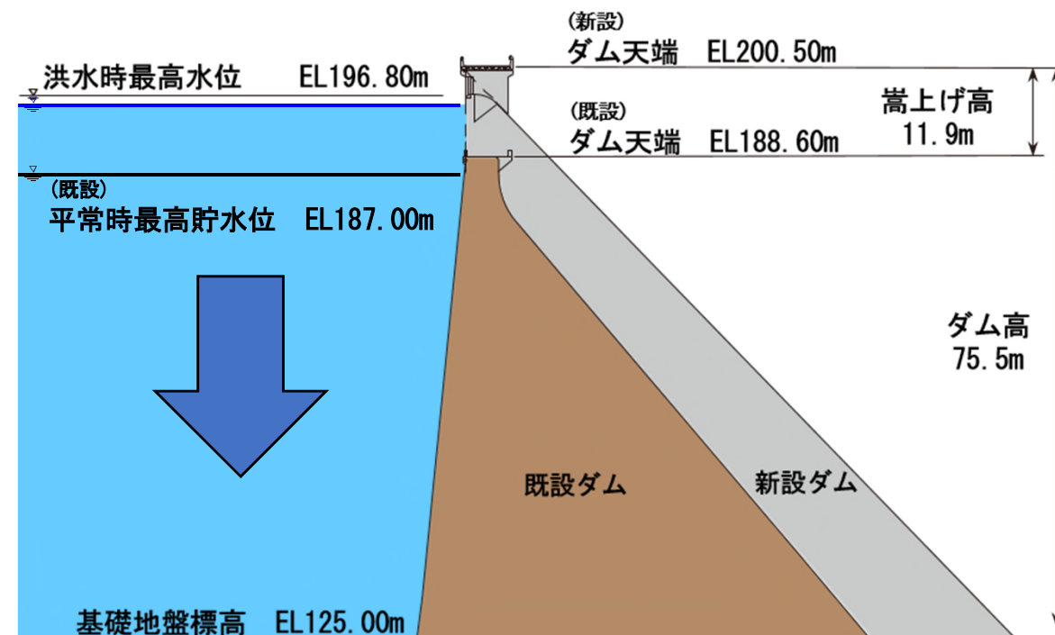
新桂沢ダム断面図
