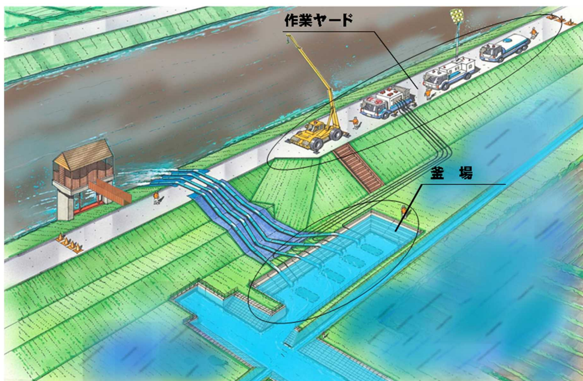
図 2-5 内水排水のイメージ図
