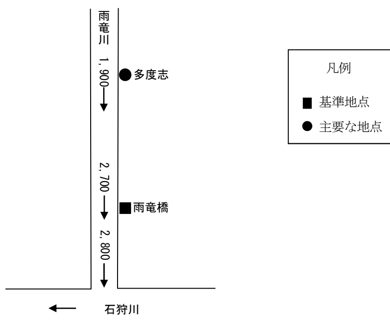
図 1-13 石狩川水系河川整備基本方針における雨竜川計画高水流量配分図（単位: \text{m}^3/\text{s} ）
