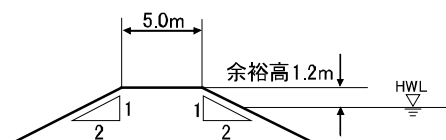
図 2-1 堤防の標準断面図
