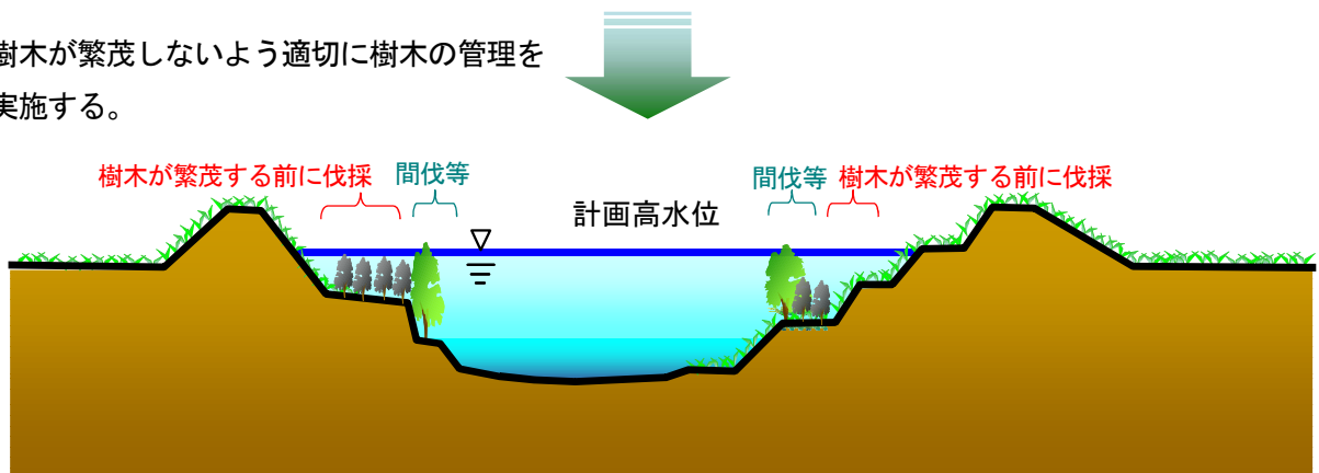
図 2-11 河道内樹木の管理イメージ図
