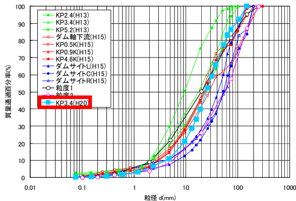
図 4.1-5 三笠ぼんべつダム 現地河床材料調査結果
