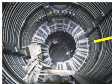
集水井工のイメージ
