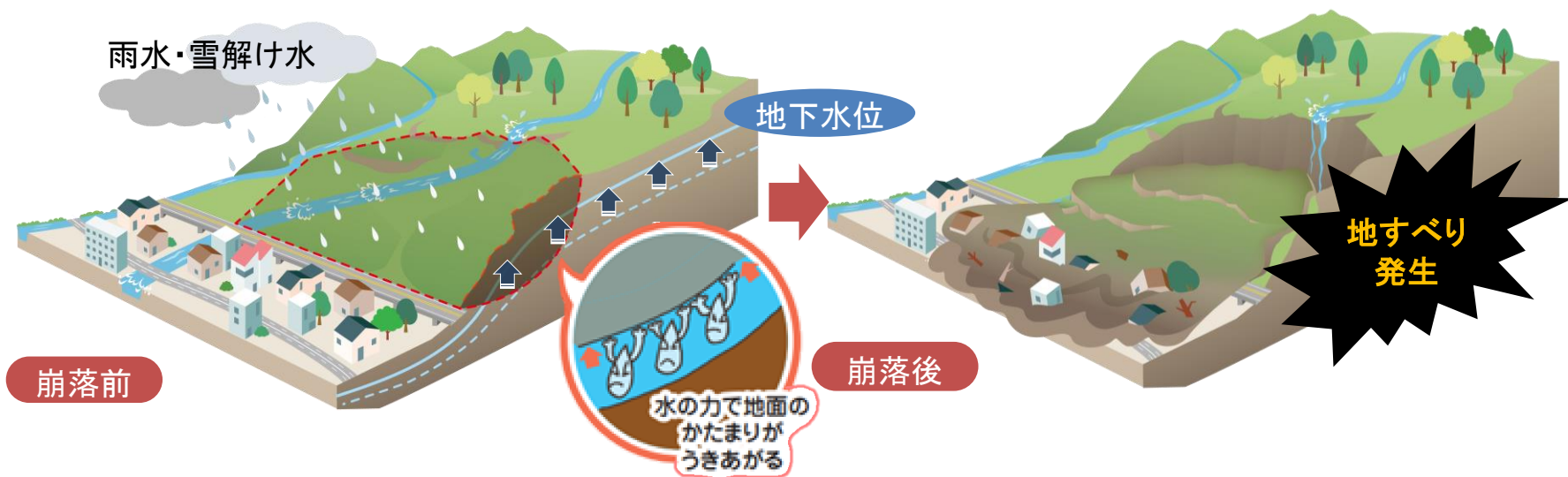
想定される地すべり災害のイメージ
