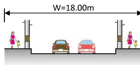
標準定規図
