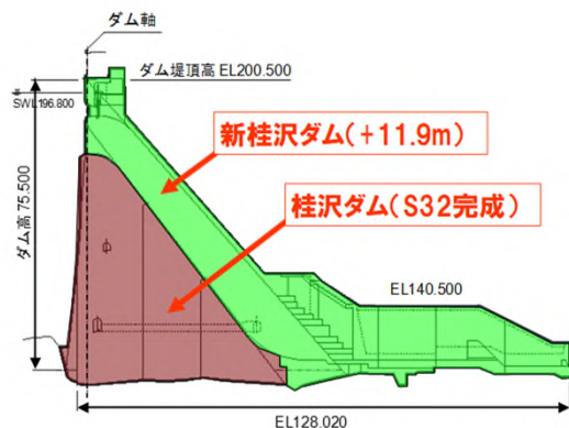
新桂沢ダムのかさ上げ
