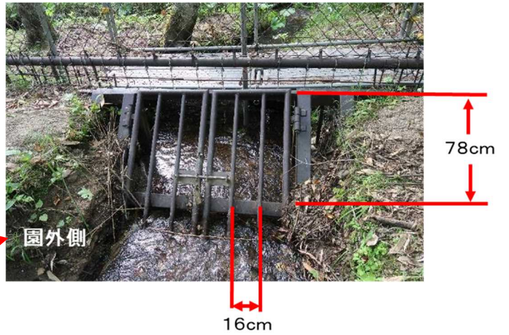
外周柵と沢の交差部のストレーナー②
