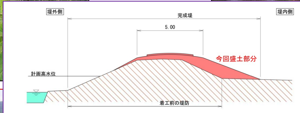
標準断面図（参考）
